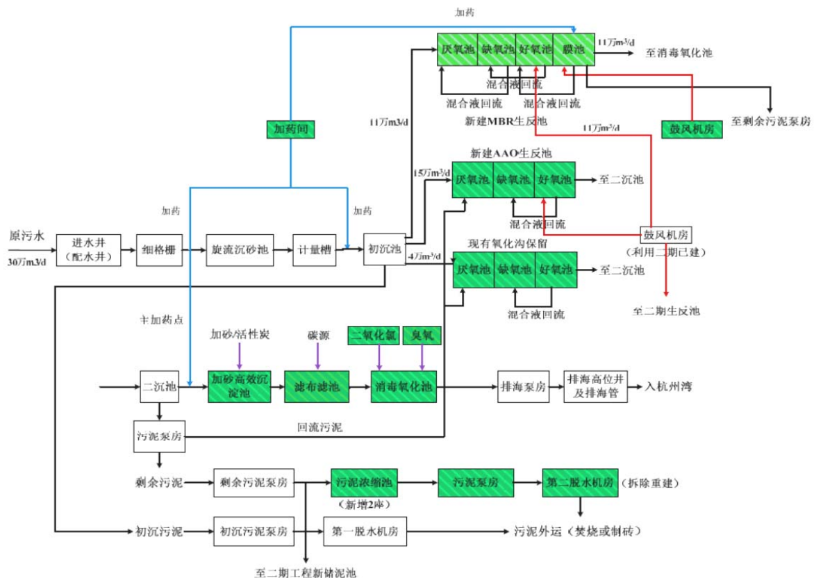
图 2-5 提标后污水处理厂一期工艺流程图
