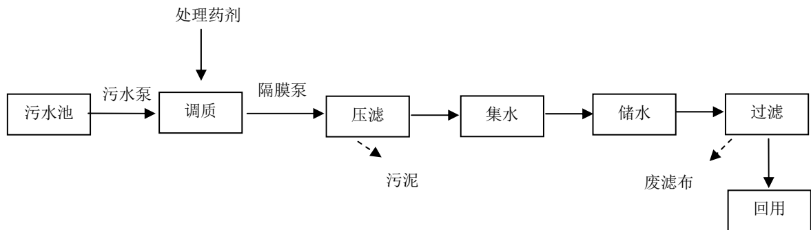
图 8-2 生产废水处理设施工艺图
