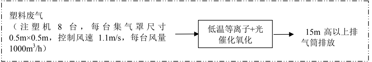
图 7-1 生产车间废气处理系统图
