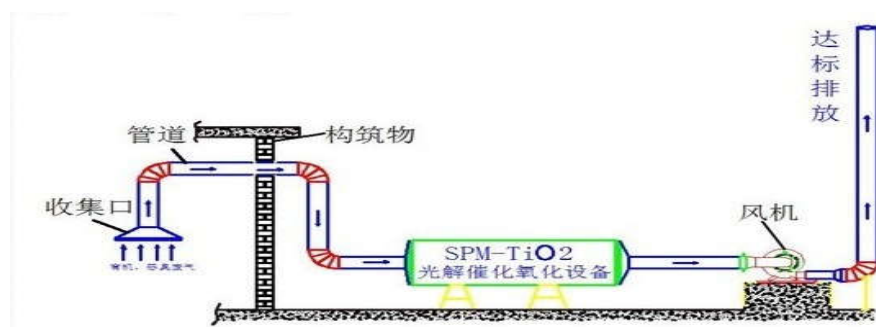
图 8-1 工艺示意图
