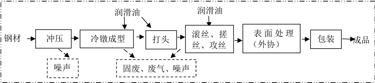
图 5-2 钢材加工生产工艺流程和产污环节图
