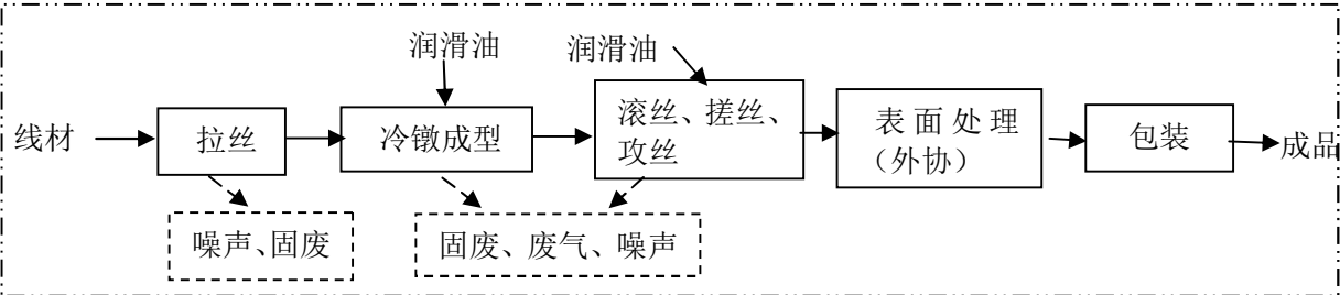
图 5-1 线材加工生产工艺流程和产污环节图
