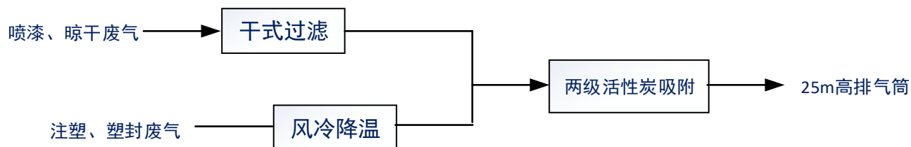
图 3-1 本项目有机废气处理系统图
